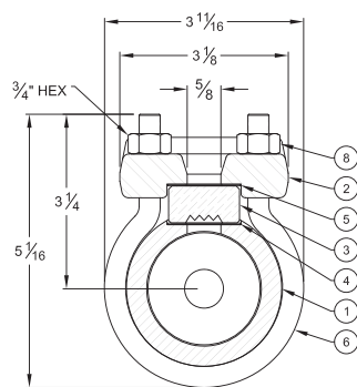
Reflex [STD. & CH]
